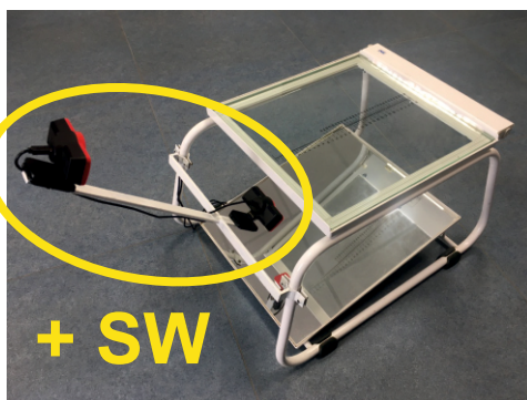
PodoCam 2.1 - 2 kamery, držák, software
